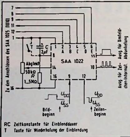
Der Anschluß des SAA 1022 an den SAA 1025.
